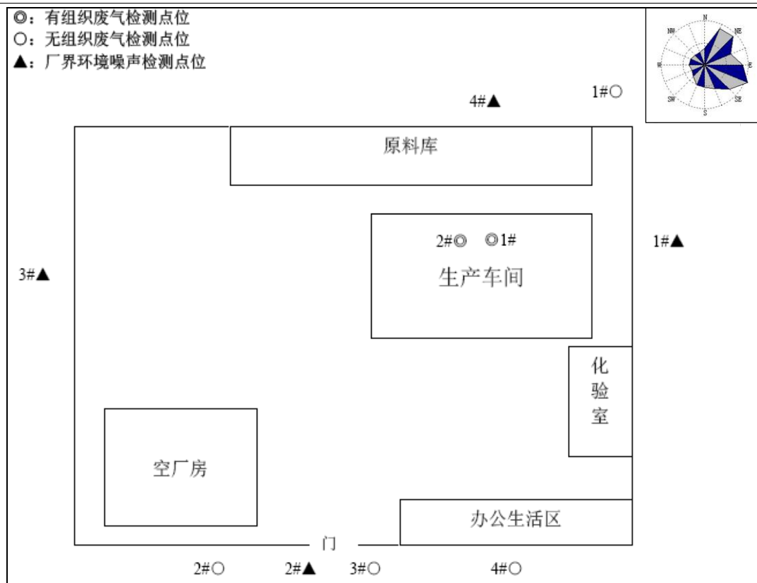
图 6-1 项目一期废气、噪声监测点位平面布设示意图
