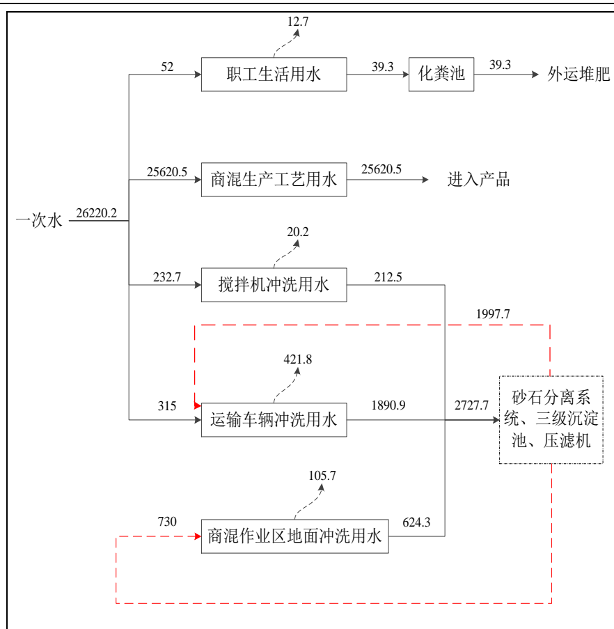
图 2-5 项目一期用水平衡图（单位：m 3 /a）
