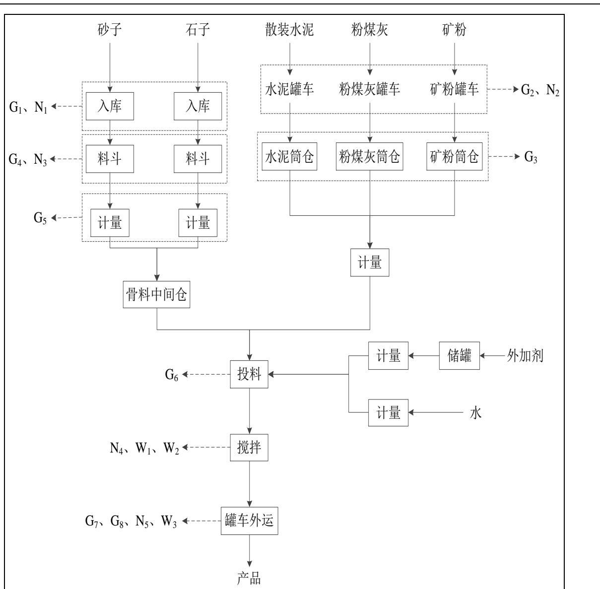
图 2-6 项目一期商品混凝土生产工艺流程及产污环节图
