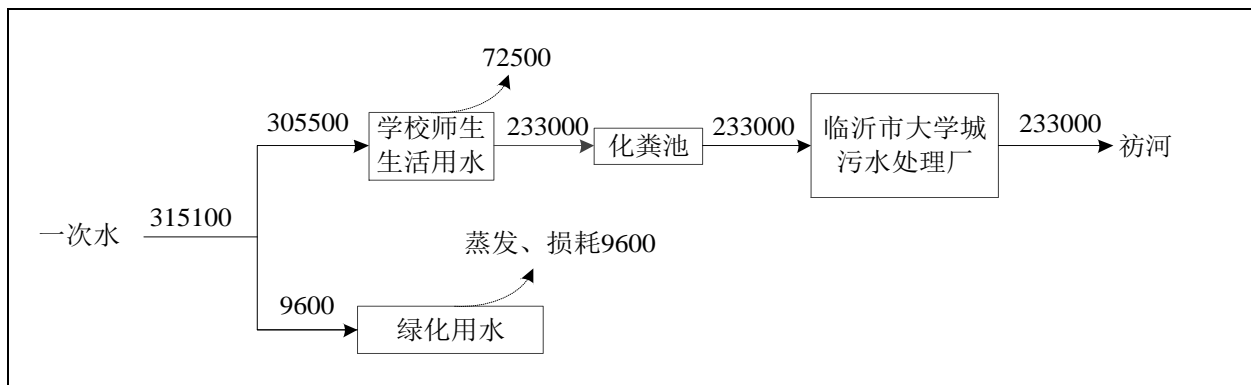
图 2-4 项目厂区用水平衡图 (单位: m 3 /a)
