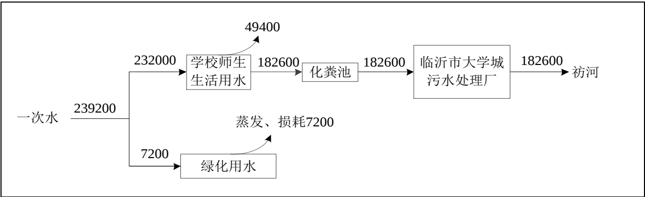
图 2-4 项目厂区用水平衡图 (单位: m 3 /a)
