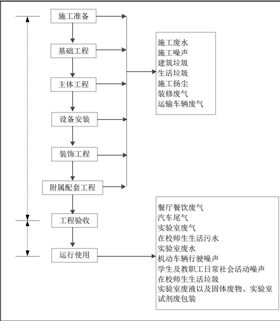
图 2-5 学校建设及运营工艺流程及产污环节图
